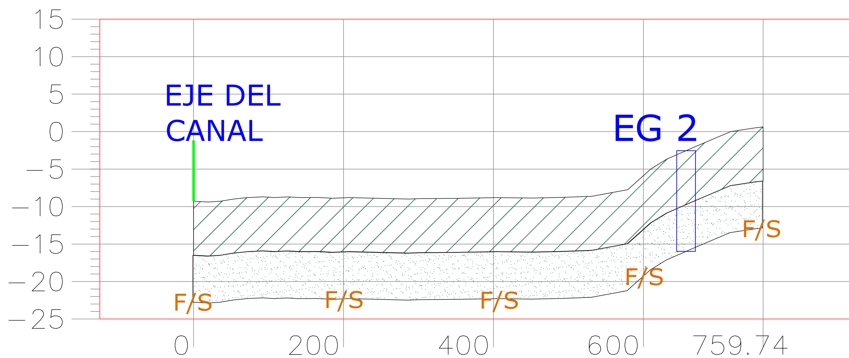
PERFIL EG2 ESCALA HORIZONTAL 1 : 1000 ESCALA VERTICAL 1 : 100
