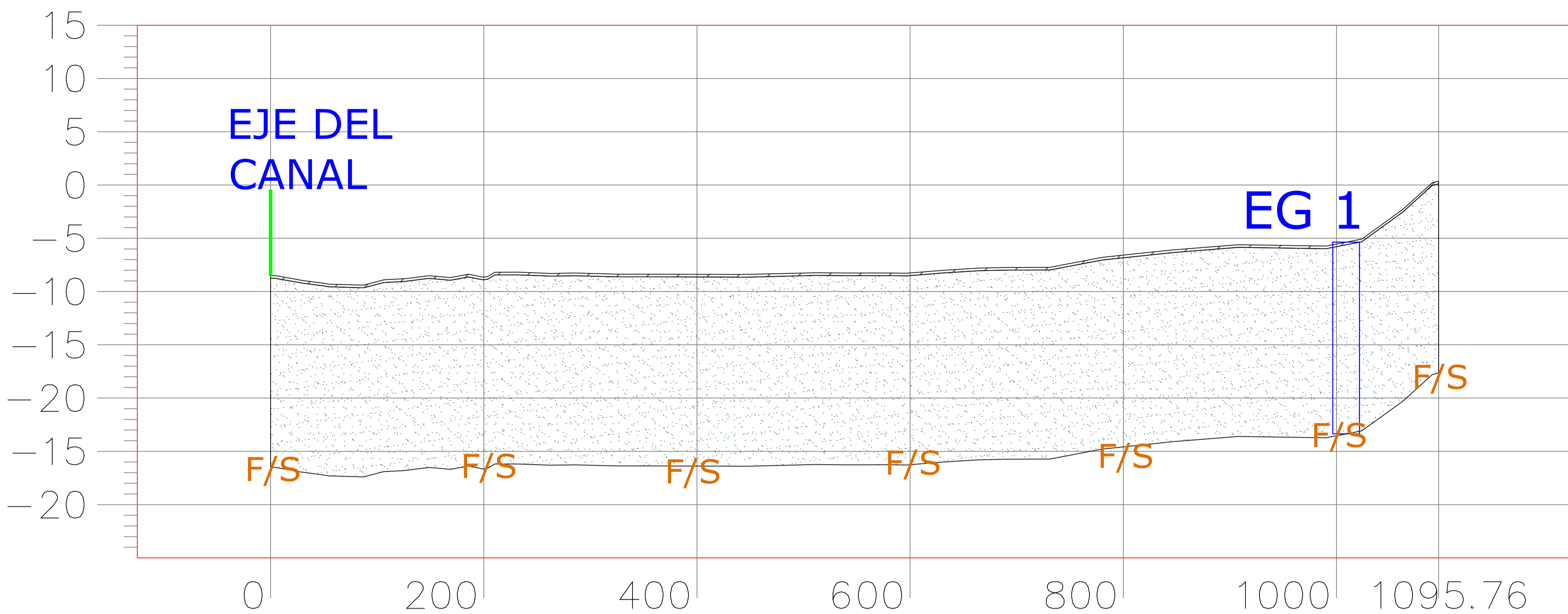
PERFIL EG1 ESCALA HORIZONTAL 1 : 1000 ESCALA VERTICAL 1 : 100
